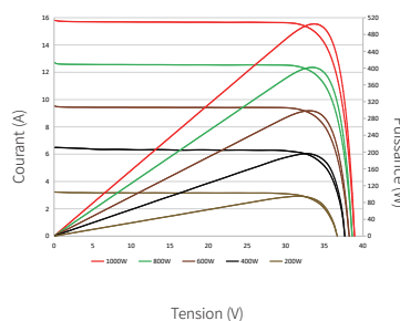
Courbes courant-tension et puissance-tension (500W)
